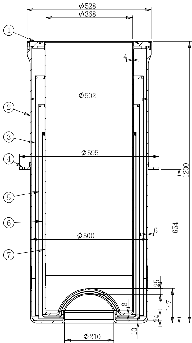
단면 A-A 배율 1 : 10
